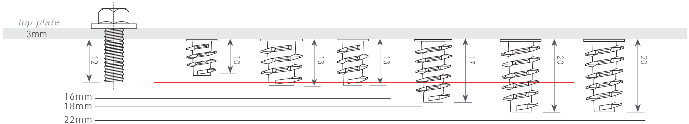
M6 x 10mm RIH1446 M8 x 13mm RIH1834 M6 x 13mm RIH1453 M6 x 17mm RIH1447 M6 x 20mm RIH1445 M8 x 20mm RIH1448
